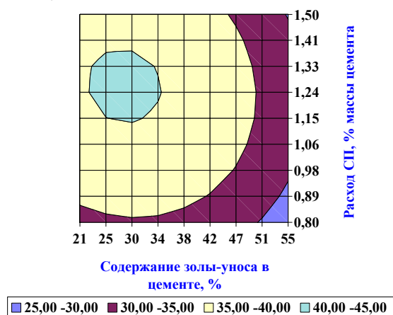
Рис. 10. Проекция поверхностей отклика зависимости прочности бетона при сжатии от типа и расхода СП при варьировании содержания золы-уноса в составе цемента.
